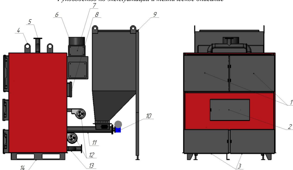
Рисунок 3 – Схема размещения составных элементов в котлах серии Eko Max DUO. 1-дверь верхняя; 2-дверь средняя; 3-дверь нижняя; 4-ухо транспортировочное; 5-труба подачи; 6-труба дымовая; 7-короб дымохода; 8-дверь дожига; 9-бункер; 10-мотор-редуктор; 11-труба топливоподачи; 12-вентилятор наддува; 13-труба обратной линии.
